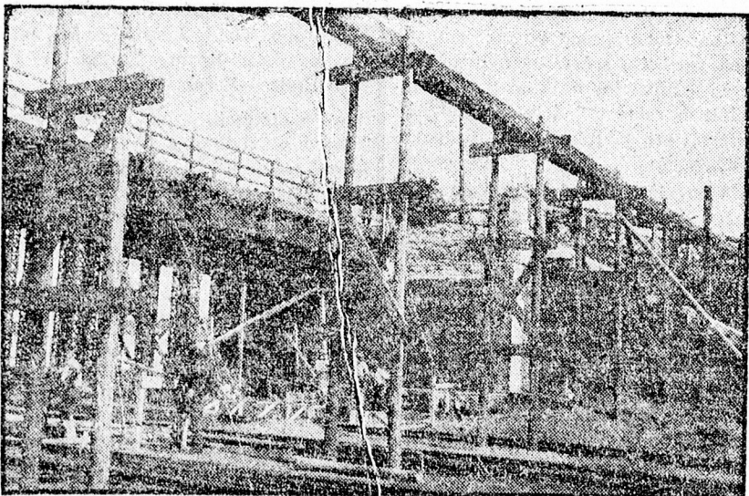
Ilyen ideiglenes állványok tartják a villany kábeleket a vasuti „nagy hid” javításánál.
