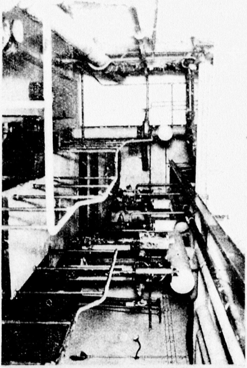
A központi fűtés kazánjainak felső hid- és csatlakoztatása.
