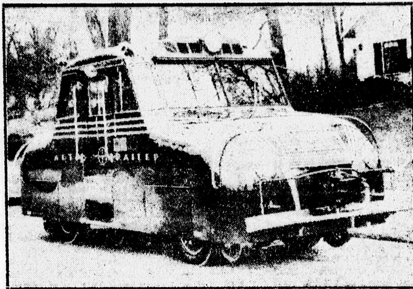
Amerikában feltaláltak egy olyan autót, mely az utcákon és a síneken egyformán használható. Ilyen autót gyárt a clevelandi vasúttársaság, egyelőre csak a pályatestek felülvizsgálására használják.
