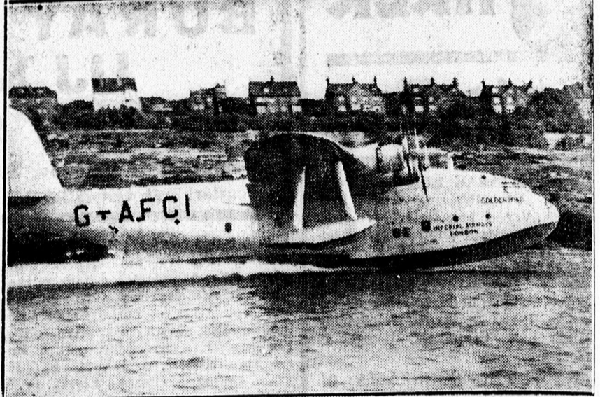
31.5 tonnás 4 motoros, óránként 320 km-es sebességgel haladó hidróplán próbautján.
