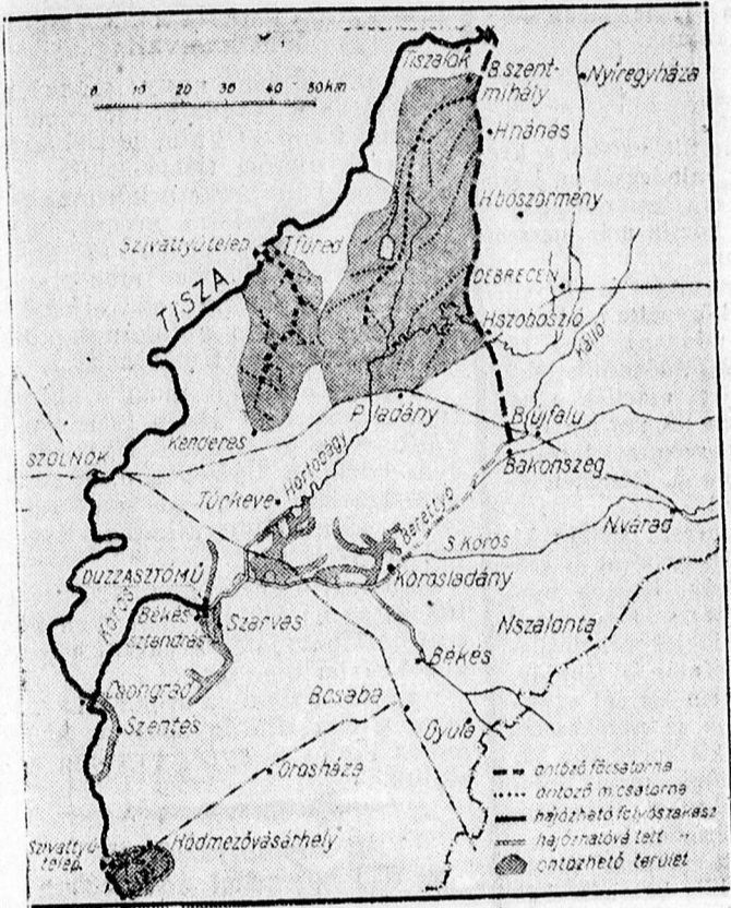
Az öntözőcsatorna térképe.
