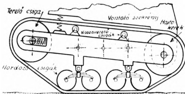
1. ábra. A hernyólánccos vontató sematikus rajza
