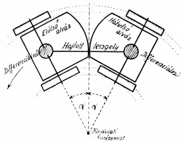
12. ábra. A Pavezi vontató fordulása
