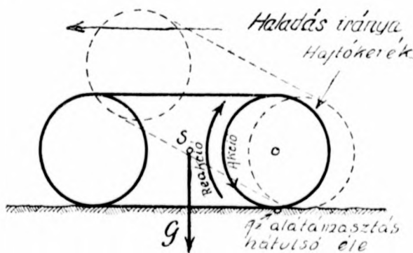
2. ábra. A hátul elhelyezett hajtókerek
