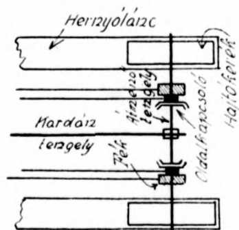
8. ábra. Munkátviteli szerkezet átfutó keresztengellyel és oldalkapcsolókkal. Sematikus rajz
