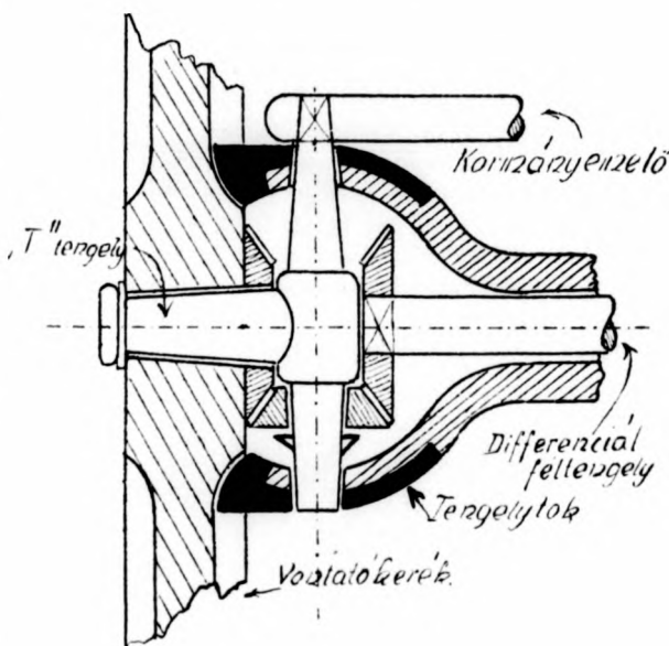
11. ábra. A kormányzott kerék meghajtásának sematikus rajza
