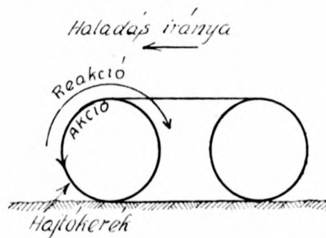
3. ábra. Az elől elhelyezett hajtókerek
