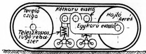
5. ábra. A Kégresse hajtás sematikus rajza
