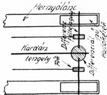
7. ábra. Munkátviteli szerkezet differenciál művel és fékekkel. Sematikus rajz
