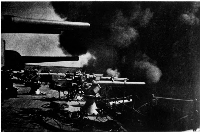
Feuernde Turmgruppe. — Tűzelő tornyok. — Grupa, koja puca sa tornja ladje. — Děla na obrněné věži za palby. — Ogień wież okrętowych. — Un grup de canoane cu turnuri trăgând focuri. — Tourelles pendant le tir. — Turrets firing.
