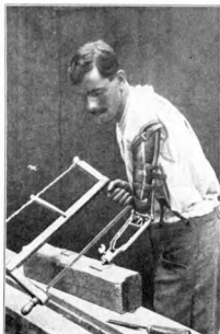
Arbeitsprothese (Eichmann) mit auswechselbaren Anhängen
