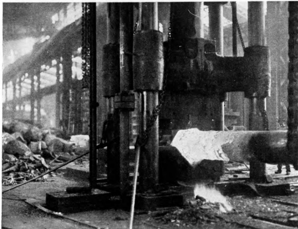
2500-Tonnen-Pressen in Funktion. — 2500 tonnaís sajtó működésben. — Preša od 2500 tona u djelovanju. — Lis majstor 2500 tun v činnosti. — 2500 tonowa prasa przy pracy. — 2500 tonowa prasa w czynności. — Pressé de 2500 tonnes en fonction. — Presse de 2500 tonnes en fonction. — A press of 2500 tons in work.
