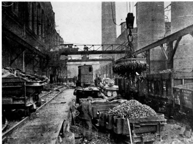
Elektro-magnetischer Kran. — Elektromagnetikus daru. — Elektro-magnetický žrád. — Elektromagnetički jeřak. — Elektro-magnetycznyj kran. — Crua electro-magnetic. — Crua electro-magnetičuo. — Electro-magnetic crua.
