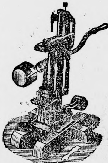
Verkorkungsmaschine.
