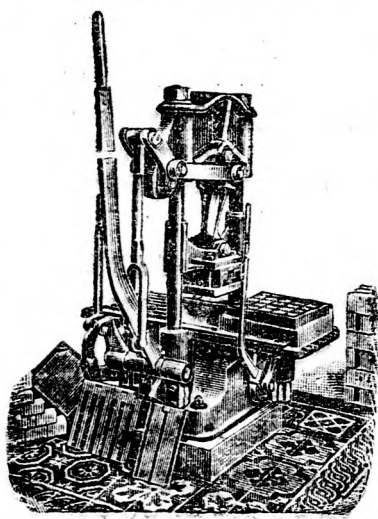
Zementplattenpresse.
