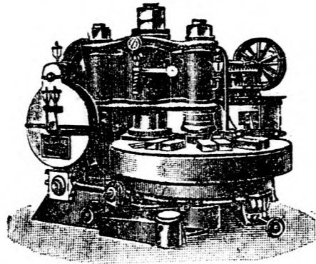
Großbetriebspresse.
