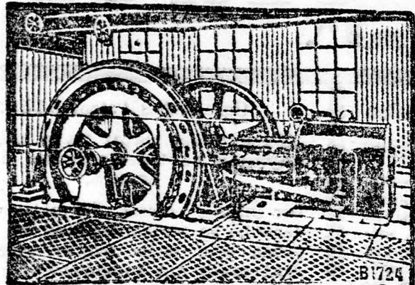
LANZ'sche Heissdampf-Ventil-Lokomobile mit direkt gekuppelter Dynamo.
