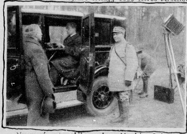
Nyomozó automobil, amelyen fényképezőgép, telefon, daktiloszkópiai osztály és trógep is van
