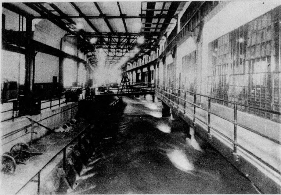
Mielőtt a Niagara folyó rohanó vize az alagútba belépne, acélrudakból készült rács tisztítja meg a hordalék kövektől
