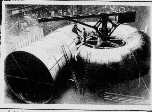
Óriási spirálturbina, amelyet most készített el egy német gyár egy irországi vízmű számára, 40.000 lóerős
