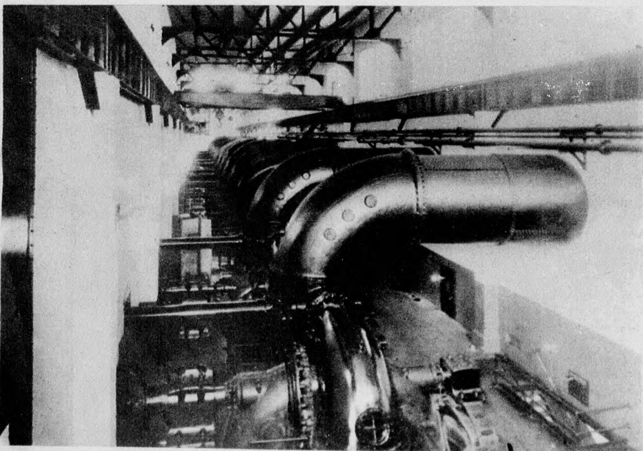
Hatalmas vascsatornák vezetik a lezuhanó vizet a szédületes sebességgel forgó turbinákhoz
