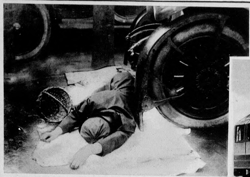
Védőkészülék autóelgázolás ellen. W. D. Ratcliff mérnök találmánya ez a készülék, amelynek szerepe, hogy megakadályozza azt, hogy az autó keresztülmenjen az elébe került áldozaton. A legsúlyosabb balesetek ugyanis abból keletkeznek, hogy a nehéz kocsik keresztülmennek az elébe került emberen és nagy súlya belső sérüléseket okoz
