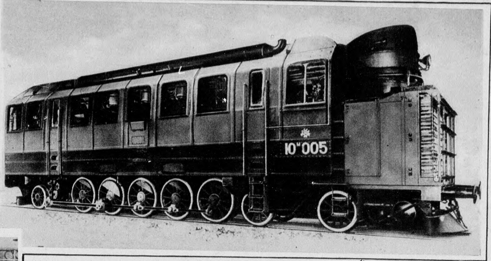
1200 lóerős új rendszerű lokomotív. A düsseldorfi Hohenzollern lokomotív-gyár nemrégben fejezte be újrendszerű lokomotívjának próbajáratát és a kísérletek a legteljesebb sikert hozták. A lokomotív hajtóerejét több, összesen 1200 lóerős kifejtésére képes Diesel-motor adja, amelyeket olajjal tartanak üzemben. Az új lokomotív nagy
