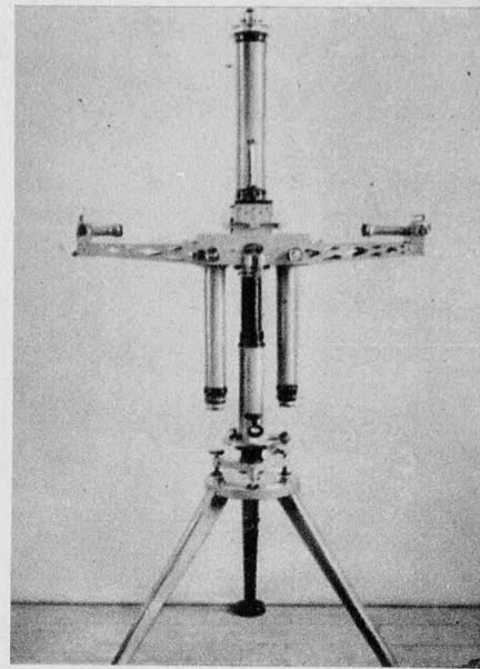
Az Eötvös-féle torziós inga
