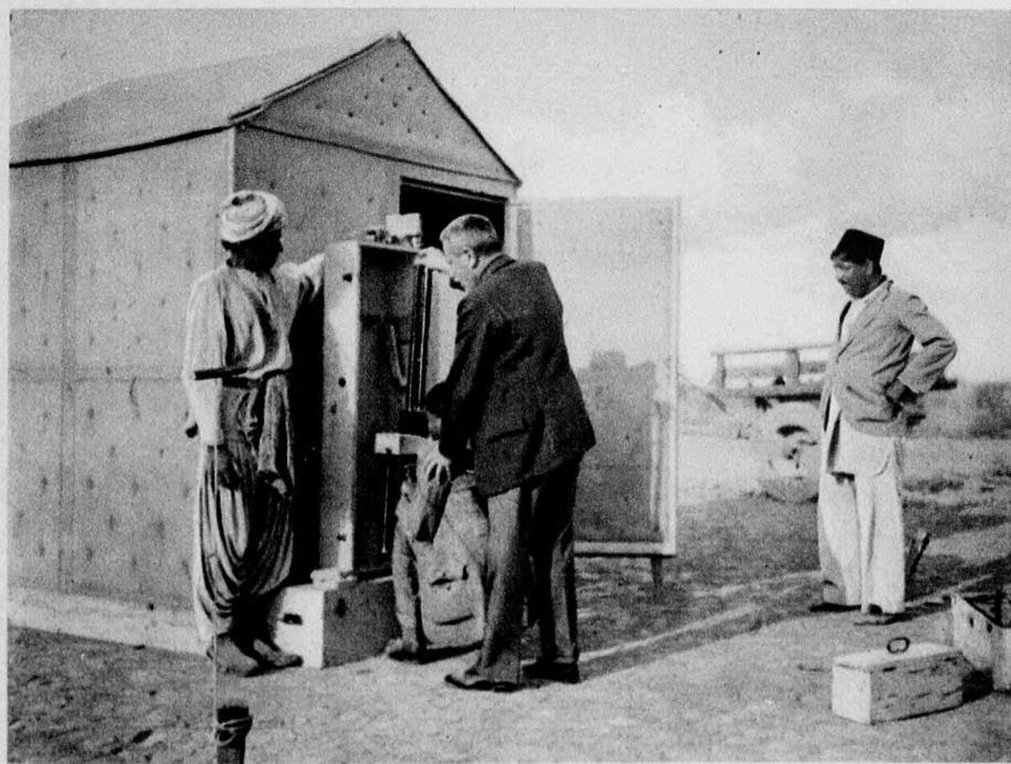
Pekár dr. hindus asszisztense segítségével a műszerház előtt kiemelt az Eötvös-műszert ládájából
