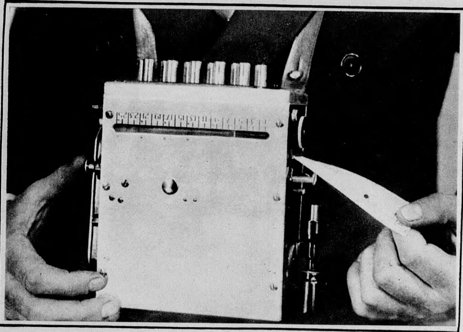
A londoni autóbuszok kalauzai ilyen hordozható jegynyomdával vannak felszerelve. Ez a kis gép a helyszínen nyomja a jegyeket, aminek az az előnye, hogy pontosan annyi jegyet nyomnak, amennyire szükségük van. A jegynyomógép egyszersmint a kalauzt is ellenőrzi és így feleslegessé válnak az ellenőrök. A berlini villamos kalauzokat is ilyen gépekkel fogják felszerelni
