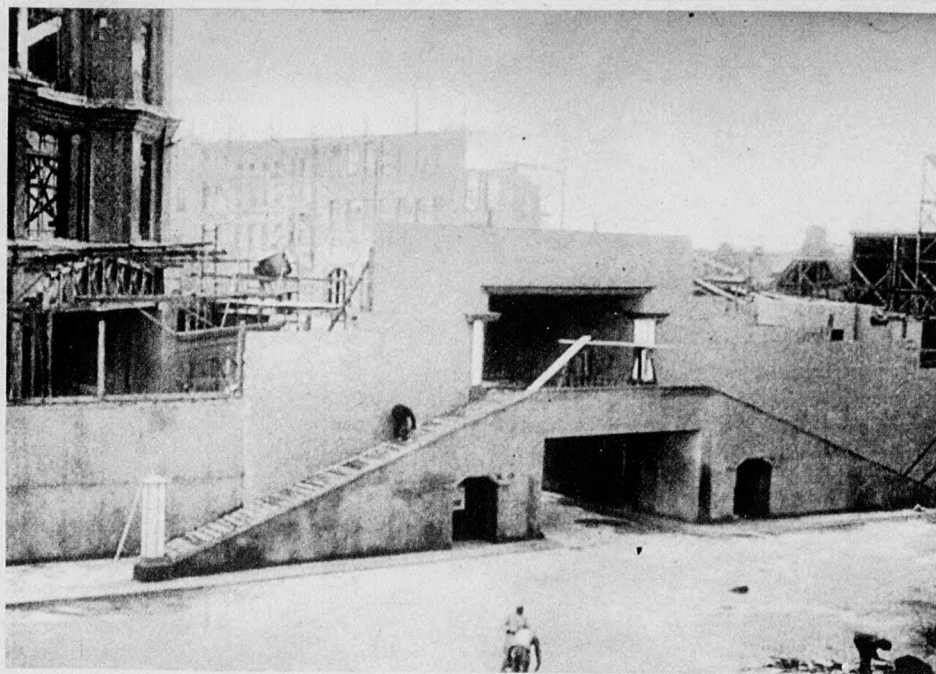
A Schüfftan-féle eljárás lényege az eredeti nagyságú alépítmény és a felépítmény kísérleti modelljének összefotografálása egy megfelelő szögben beállított tükrök segítségével
