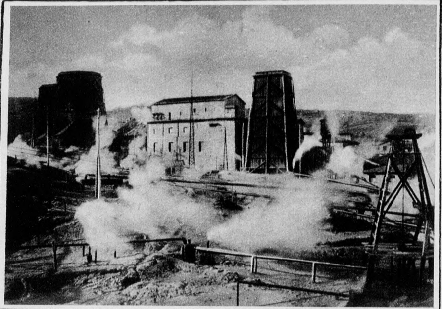
Az olaszországi Volterra közelében a földben rejlő vulkánikus erőket használják ki és ezek a forró gőzök sok ezer lóerőnyi villamoserőt szolgáltatnak
