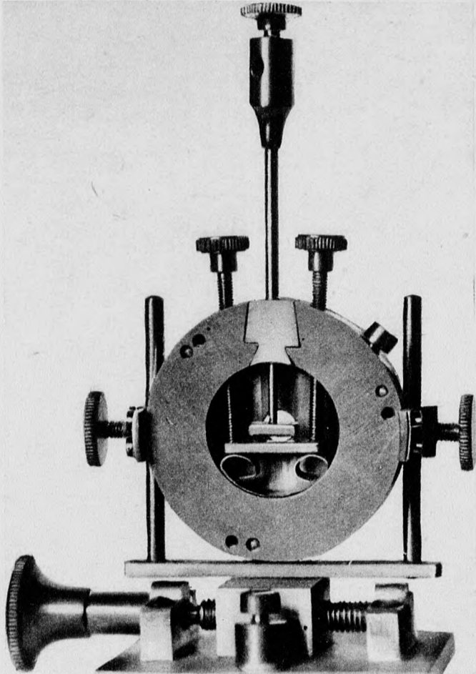
A fényérzékeny foto-cella. A karolus-féle képtávíró legfontosabb alkatrésze
