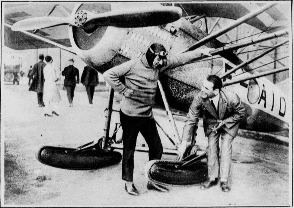
A repülőgépek leszállásának megkönnyítésére egy francia mérnök új szerkezetet talált ki, amely a törékeny kerekeket helyettesíti. A Le Bourget-i repülőtéren most próbálják ki a traktorszerű láncszerkezetet
