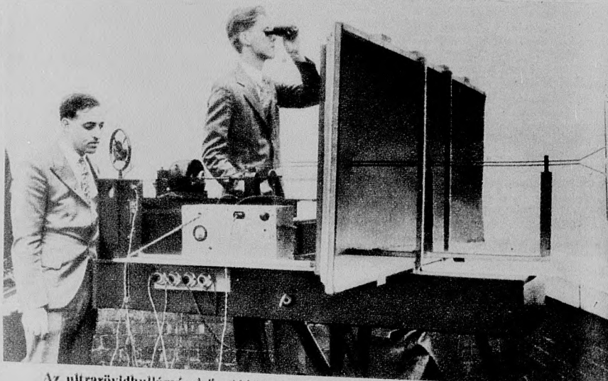
Az ultrarövidhullámú első adóállomás. A felfedezés még kísérleti állapotban. A parabolikus antenna jól látható
