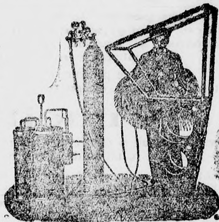
(Ko 199—126)
