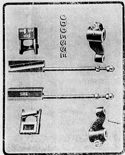
Fig. 3. Lose Steuerungsteile der Odessa-Pumpe.
