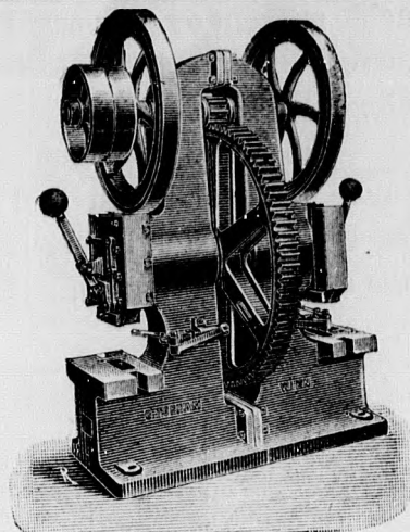
Doppelte Excenterpresse.
