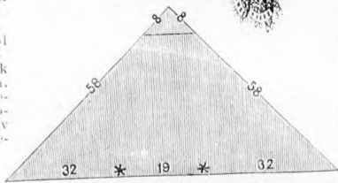
60. sz. Az 59. kép szabásrajza.
