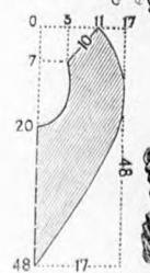
29. sz. Pántgallér. Ehhez a 30. sz. rajz
