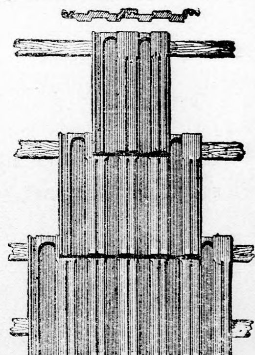
Zsombolyai gyártmány. Szab. biztonsági préselt átfedő cserep 253.
