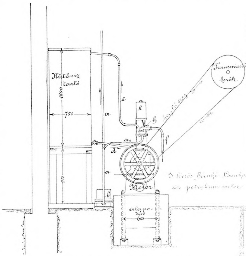
Bánki-Csonka-féle petrolum-motor.
