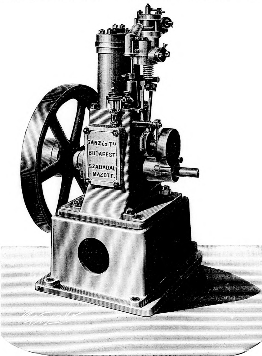
Bánki-Csonka-féle petroleum-motor.
