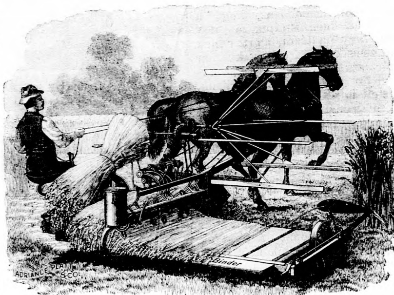
3. ábra. „Adriance” kévekötkő aratógép.
