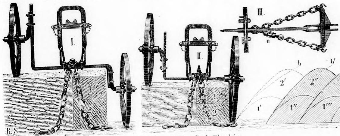
2. ábra. Önvezető készülék a Sack-féle ekén.
