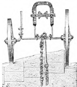
6. ábra. Taligabeállítás a Sack-féle ekénél bogárhátas szántásnál.
