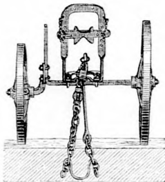
4. ábra. Taligabeállítás a Sack-féle ekénél szántásnál.
