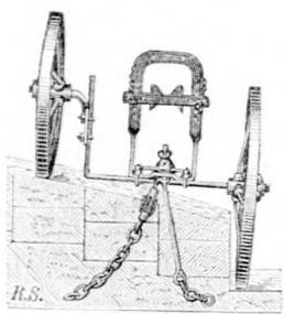
5. ábra. Taligabeállítás a Sack-féle ekénél bogárhátas szántásnál.
