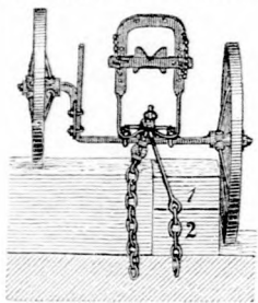
3. ábra. Taligabeállítás a Sack-féle ekénél szántásnál.
