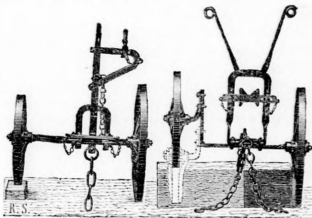
1. ábra. A Sack-féle eketaliga kerekének emelése a tengely függélyes nyulványán. (Jobboldali kép.)
