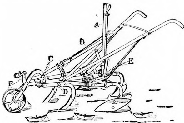
3. ábra. Osborne-féle „Columbia“ fogatos kapálógép.
