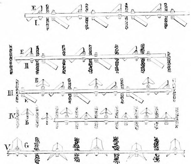
5. ábra. Kapaállítások a Sack-féle egyszerű többsoros kapálógépen.
