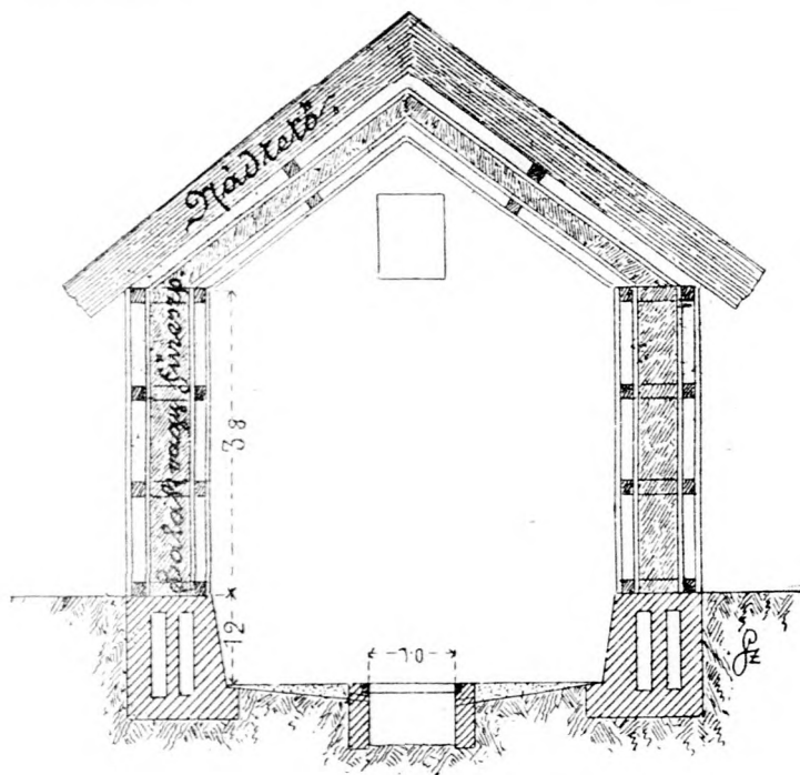
Egyszerű jégverem metszete.
