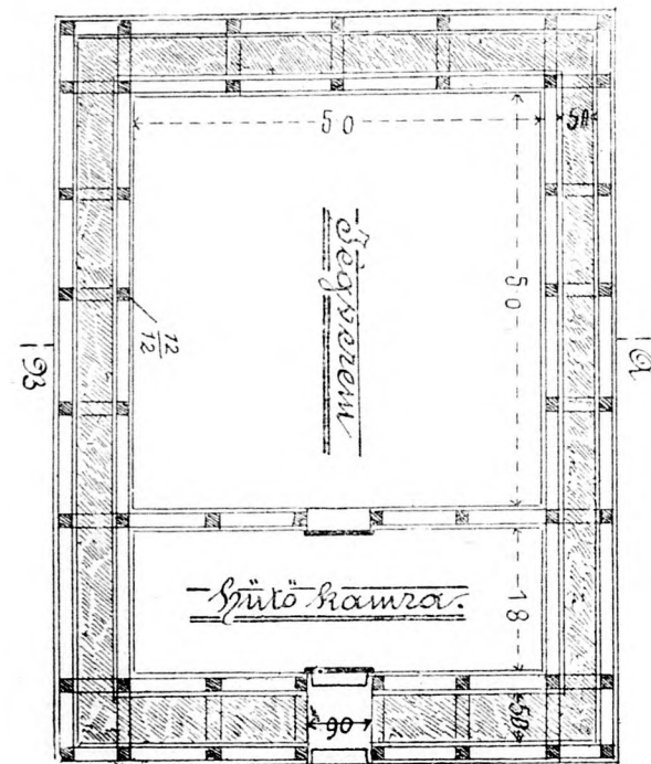
Egyszerű jégverem alaprajza.
