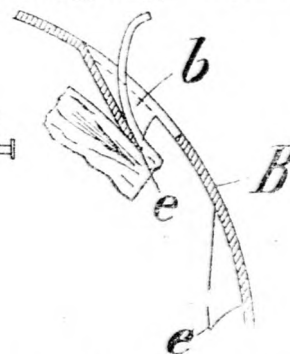
2. sz. ábra. A Göndör-féle répavágó metszőköpenyének egy kése.
