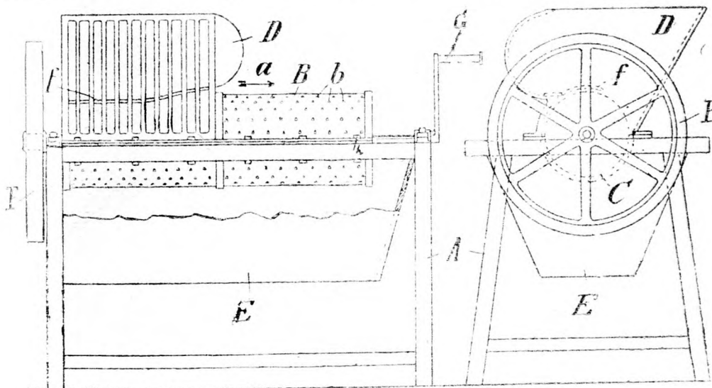
3. sz. ábra. A Göndör-féle répavágógép.
