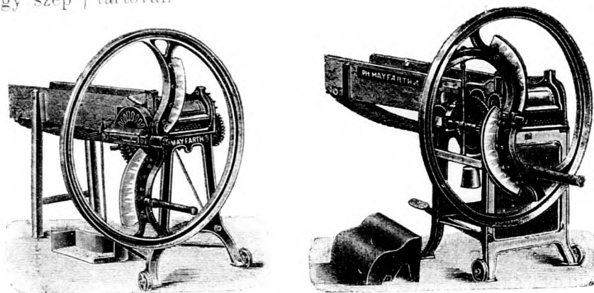
Könnyűhajtású szeckavágógépek.
