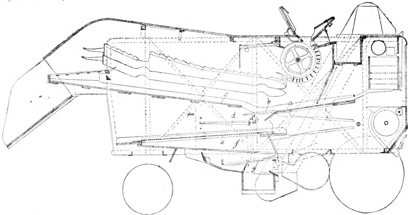
Czárán-féle kettős törekrázó.
