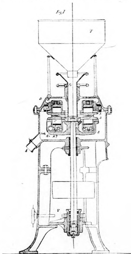
»Ottynia« daráló és őrlőmalom szerkezete.
