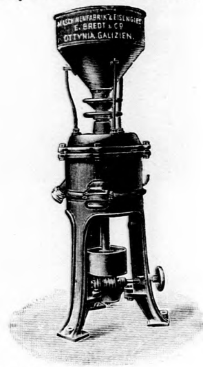
»Ottynia« daráló és őrlő malom.
