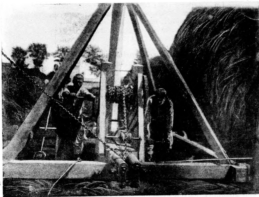
A gólya emelő-szerkezete.
