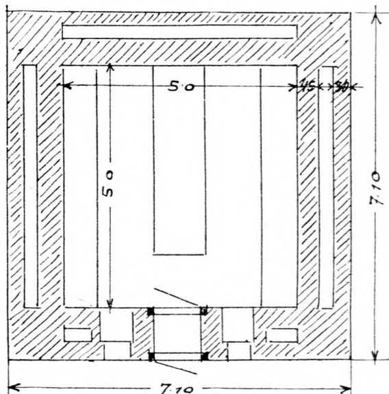
Gyümölcstartó kamra alapja.
