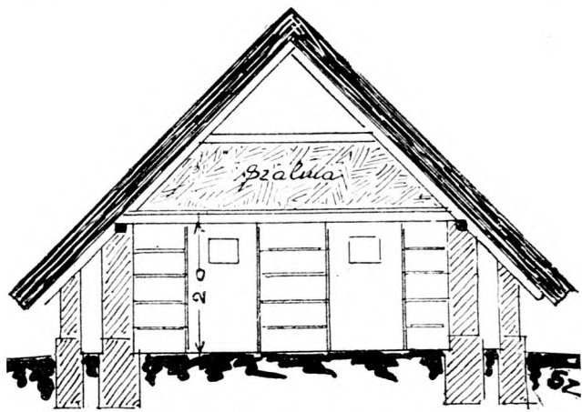
Gyümölcstartó kamra keresztmetszete.
