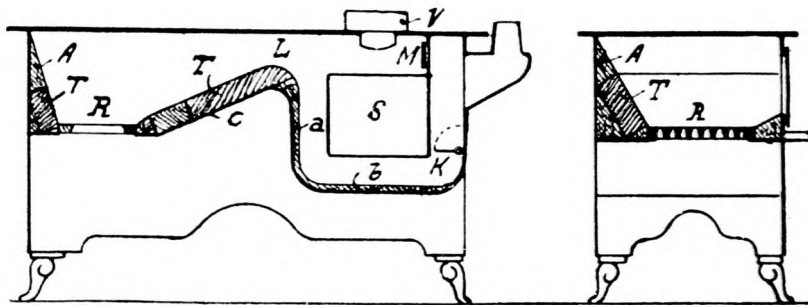
Munkácsy-féle takaréktüzhely hosszmetsete és keresztmetsete.
