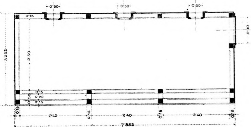
Nyílt méhes alaprajza.
