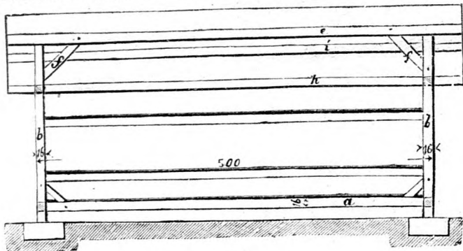
Hosszmetszet.
