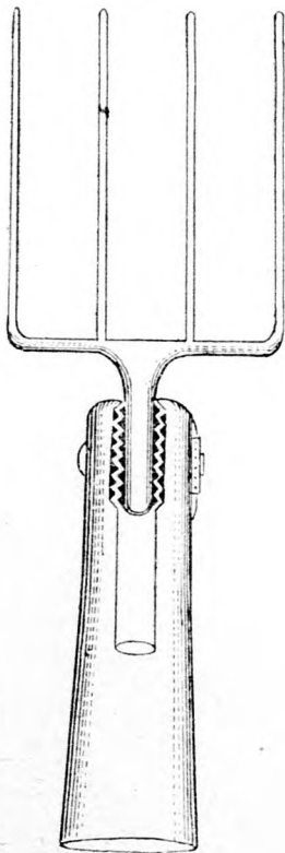
Az egytetemes talajmivelő eszköz villához alkalmazva. (Balról a nyakszorítóval ellátott szénavilla hüvelyébe téve látható míg jobbról ugyanez a ferde pontozott vonal irányában állítva mint villa, vízszintes helyzetben mint trágyahúzó kapa vagy gereblye van bemutatva.)
