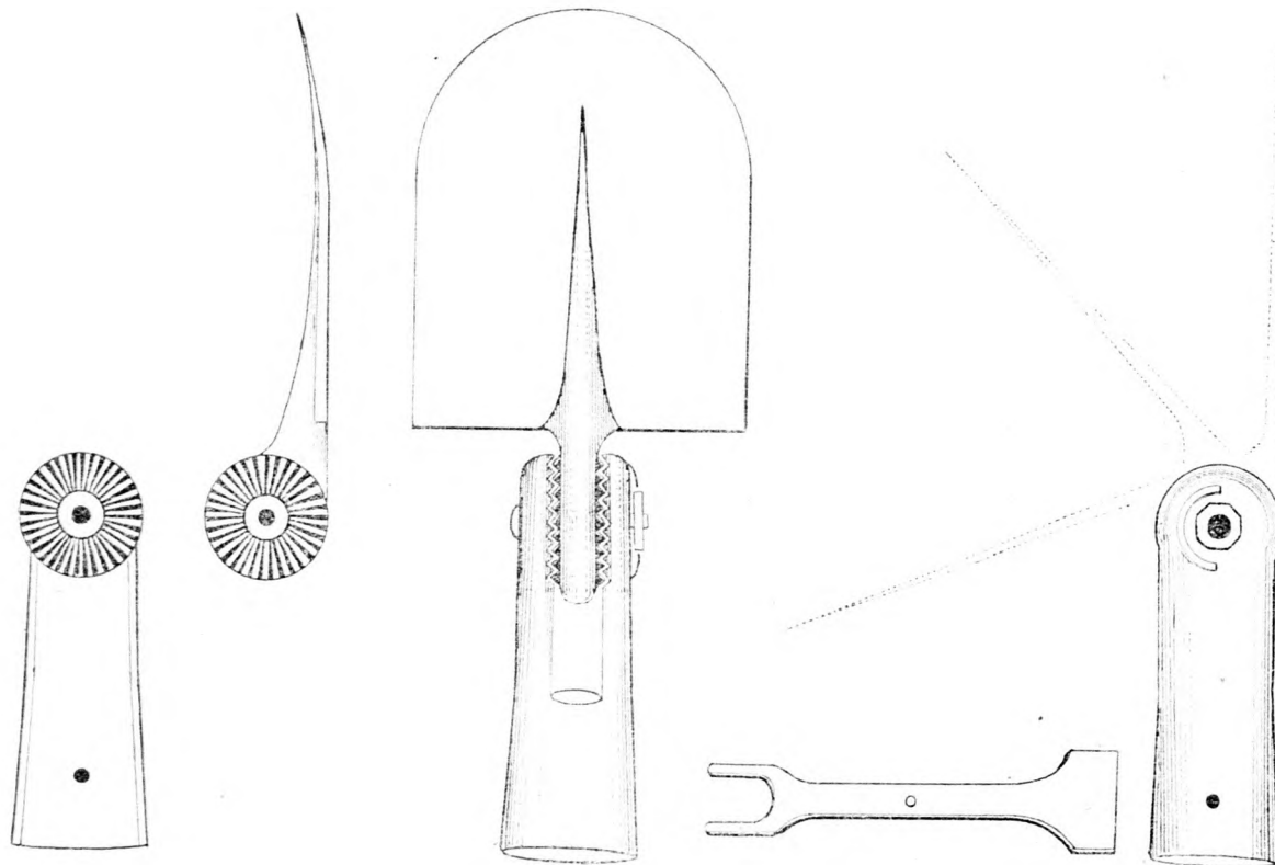
Az egyetemes talajmivelő eszköz ásóhoz alkalmazva. (A baloldali rajz a nyaktárcsát hosszmetében mutatja, a második kép a nyaktárcsával ellátott ásót, míg a harmadik e kettőt összeállítva előnézetben tárja elénk. A negyedik kép a csavarkulesot mutatja be, mely egyúttal az ásó tisztítására is szolgál. Az utolsó rajzon a pontozott vonalak függőleges helyzetben az ásót, középső állásban ezt mint lapátot és a harmadik lefelé hajtva mint kapát mutatják be.)
