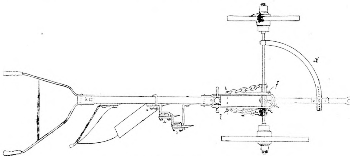
Magyar András ekéje felülnézetben.
