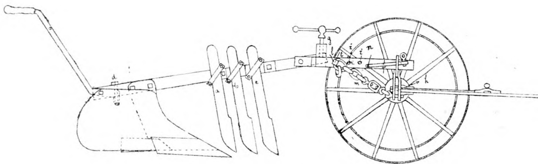
Magyar András ekéje oldalnézetben.
