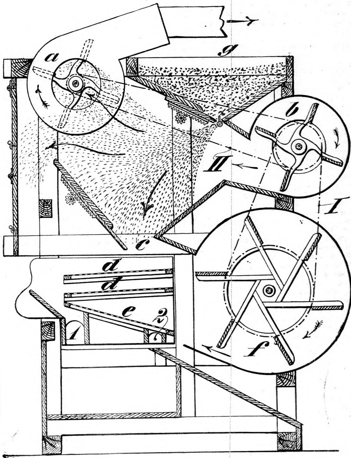
A Kalmár Zs.-féle „Non plus Ultra“ kettős terménytisztító gép.
