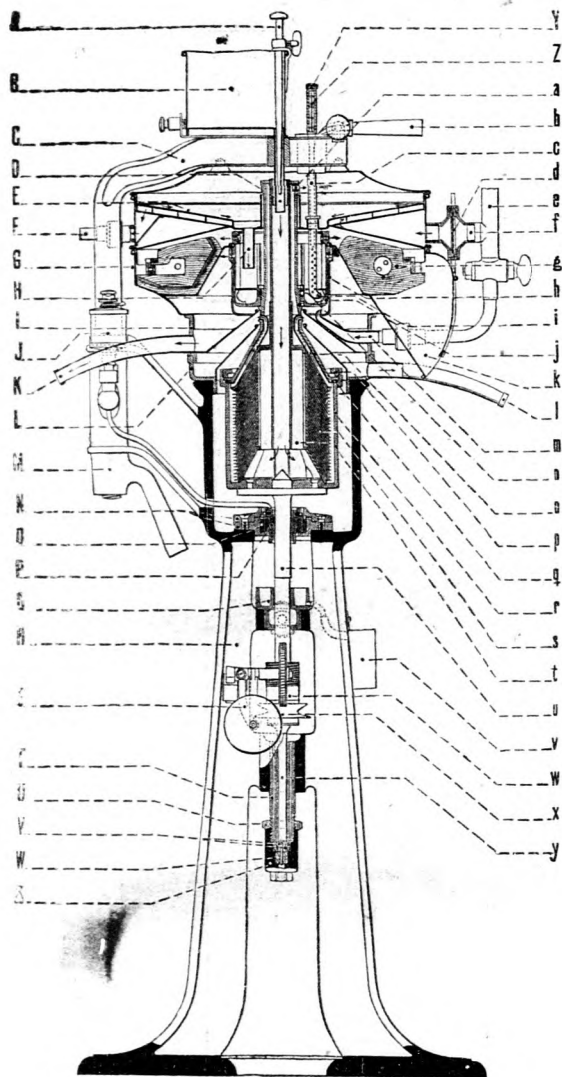
A „Radiátor“-gép keresztmetszete.
