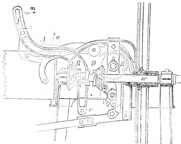
Védőkészülék, kezeknek a szecs kavágóba való behuzása ellen. (Umráth és Társától Budapesten.)
