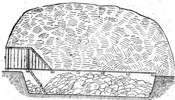
Házilag előállított jégverem keresztmetszete.
