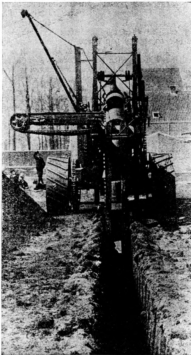
Az alagsövező gép munkája.
