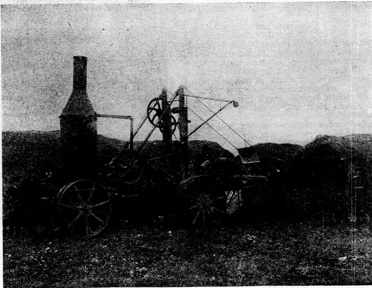
Az „Auróra” alagsövező gép munkába beállítva.
