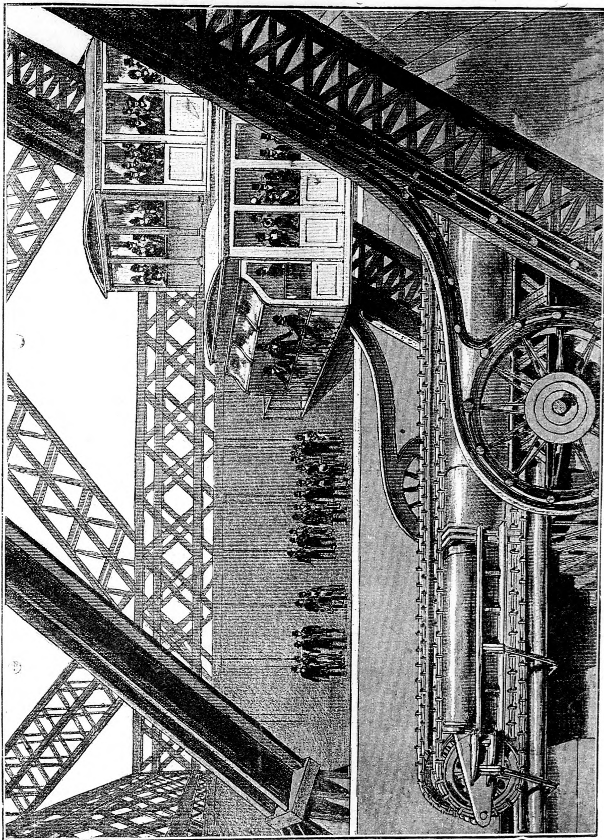
A párisi Eiffel-torony felhúzó gépe.
