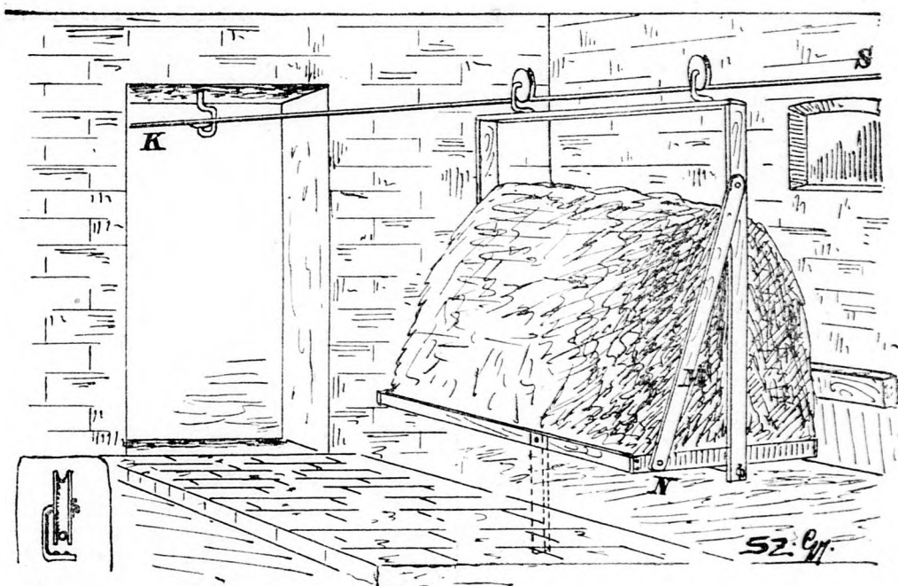
A függő trágyaköcsi szerkezete.
